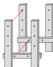
Dwarsbalken inwendig (loopvlak korter dan reling)
