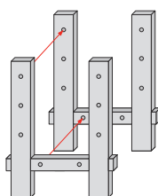
Dwarsbalken doorlopend (touwen gelijke lengte)
