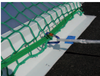
Aanslagpunt voor karabijnhaak
