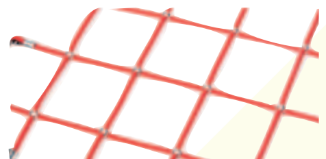
Câble Hercule 6 torons Ø 18 mm avec bille de croisement en aluminium
